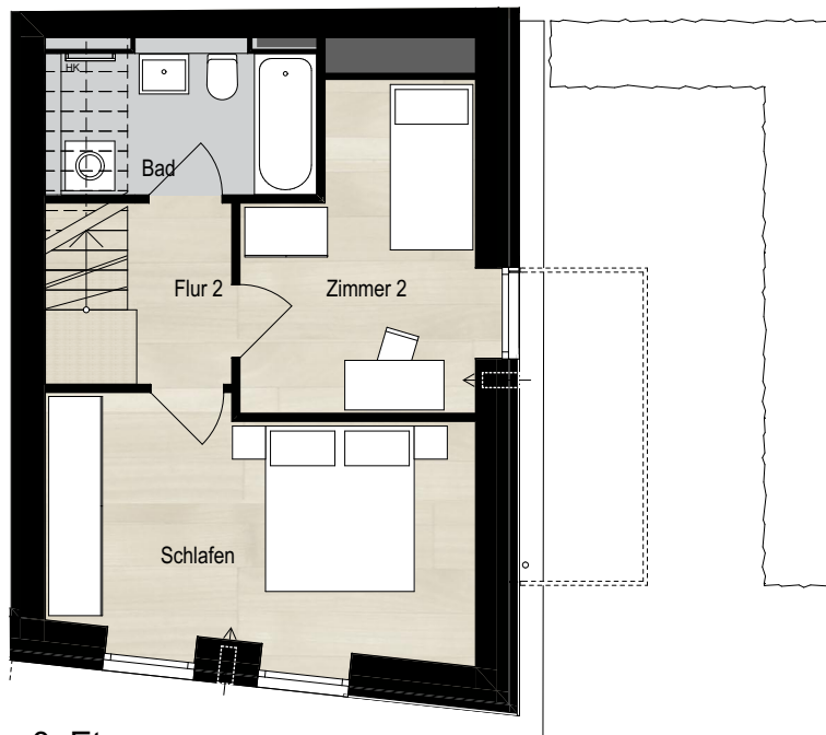
0. Etage
